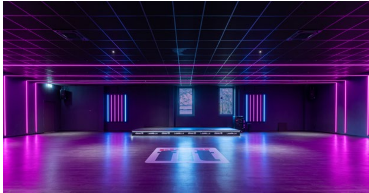
Bild links: Podestbeleuchtung | Effektbeleuchtung an Trasse Bilder rechts: Lineare Lichtgestaltung „Wand-Decke“, Maßanfertigung sowie Stripes (neben Bühne), jeweils mit „Sound-to-Light“ Effekten
