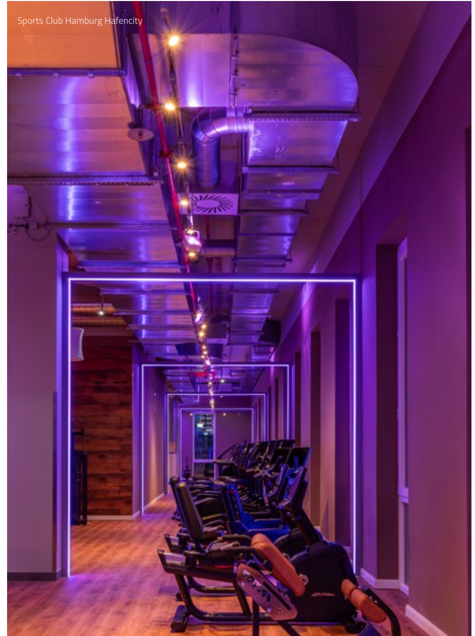
Sports Club Hamburg Hafencity Bild oben: Lineare Lichtgestaltung „Torbogen“, Maßanfertigung | Schienenspots und Effektlichter Bild rechts: Lineares Licht „Karree groß downlight“, Maßanfertigung | Lichtschienen mit Spots & Effektbeleuchtung
